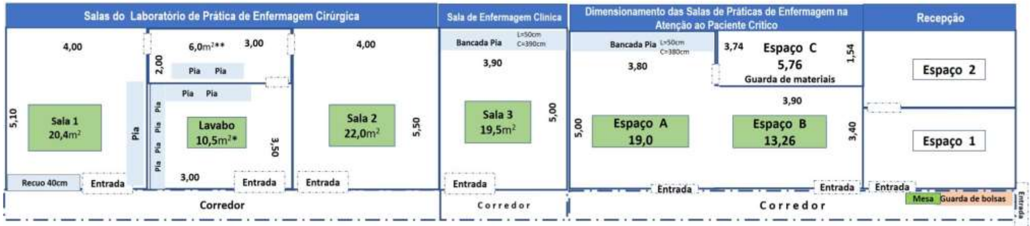
Figura 2. Dimensionamento dos Ambientes do Laboratório 2 (m 2 )
